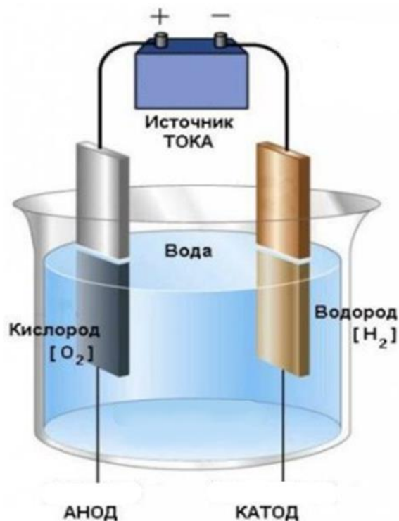
Схема электролиза
